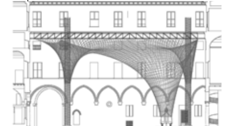
sezione della copertura rimovibile
